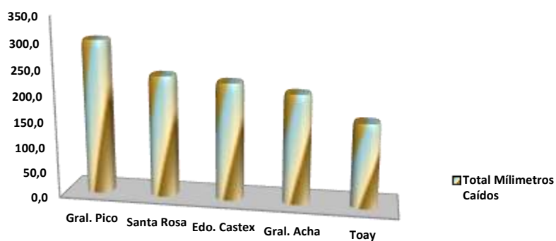
Acumulado de Precipitaciones - Total Provincial y principales localidades. 4º Trimestre 2015.
