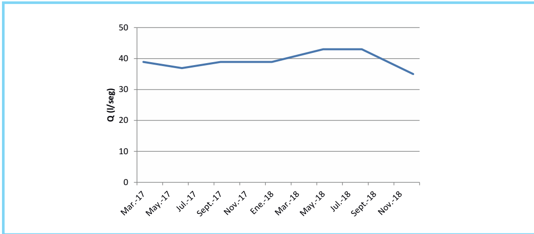
Gráfico 7. Caudal de Manantial Buta Ranquil Norte. Periodo 2017-2018.
