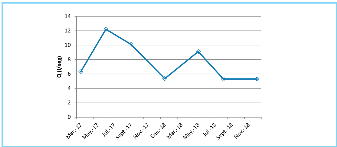
Gráfico 5. Caudal de Manantial Agua de Torres. Periodo 2017-2018.
