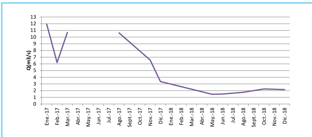
Gráfico 2. Caudal río V. Periodo 2017-2018.
