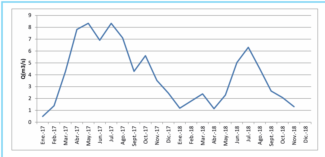
Gráfico 1. Caudal río Atuel. Periodo 2017-2018.
