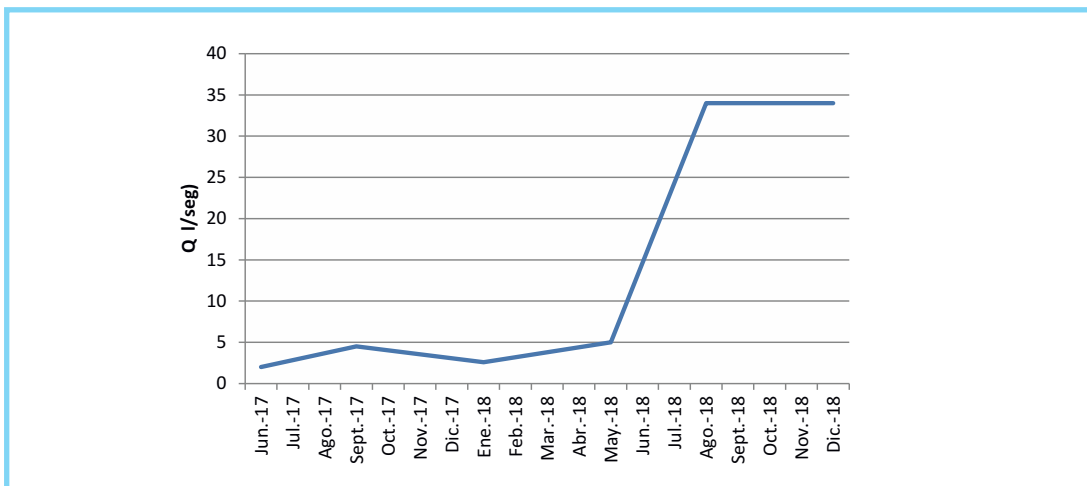
Gráfico 8. Caudal de Manantial Los Carrizales Sur. Periodo 2017-2018.
