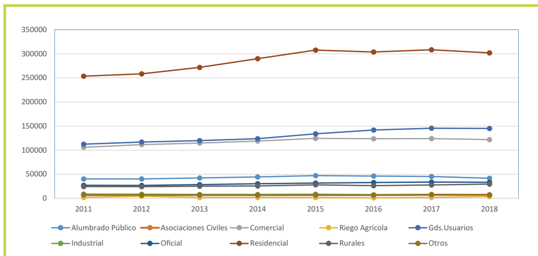
Gráfico 60. Consumo de Energía Eléctrica por Categoría (en miles kWh). La Pampa. Período 2011-2018.
