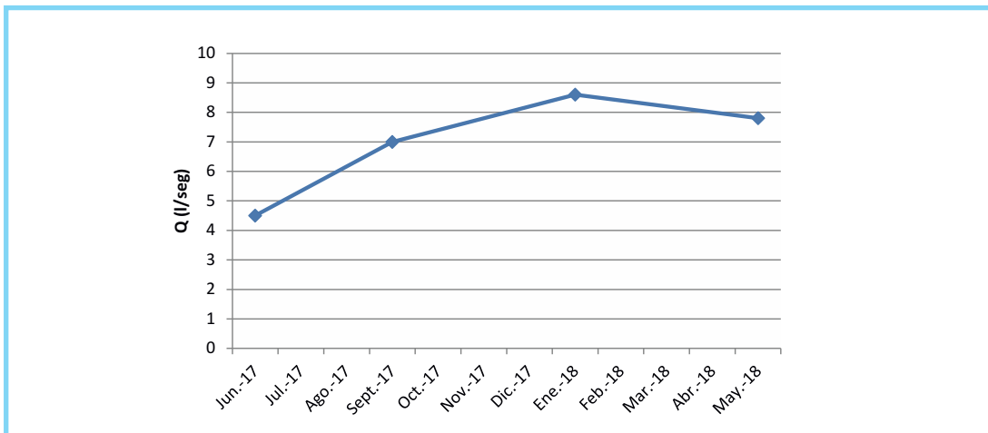
Gráfico 10. Caudal de Manantial La Copelina. Periodo 2017-2018.
