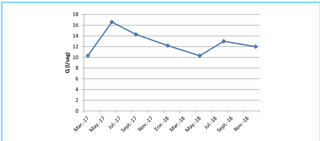
Gráfico 9. Caudal de Manantial Los Carrizales Norte. Periodo 2017-2018.
